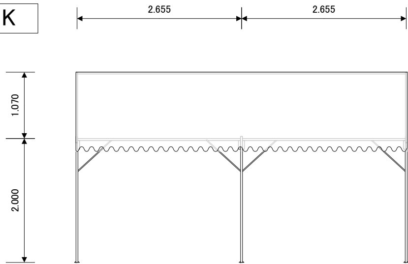
正面図
